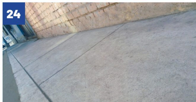
VEREDAS CALLE C ASOC. DE VIV. EL OLIVAR DE VITARTE
